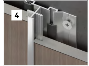
4 外包压条节点
