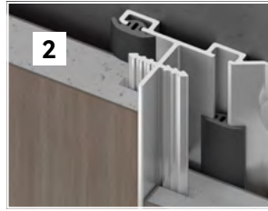
2 十字平缝压条节点
