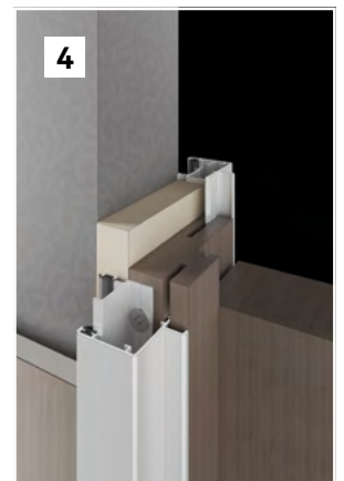
4 哑口套收口节点图
