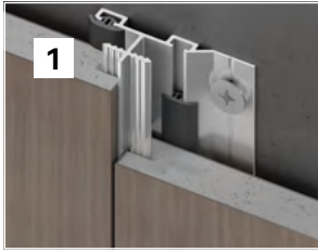
1 十字凹缝压条节点
