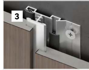
3 水缝压条节点
